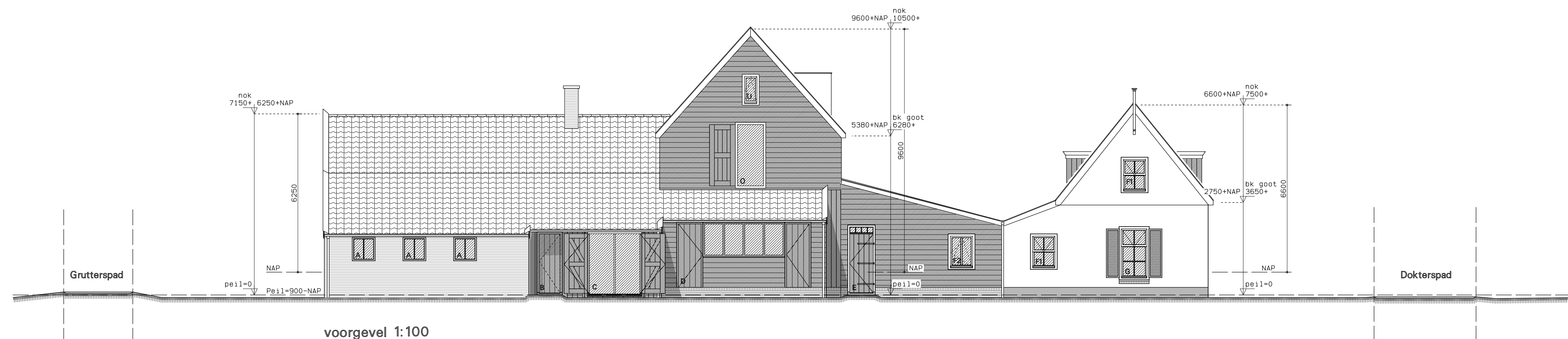
voorgevel 1:100 aanzicht vanaf Nieuwland nieuwe situatie
