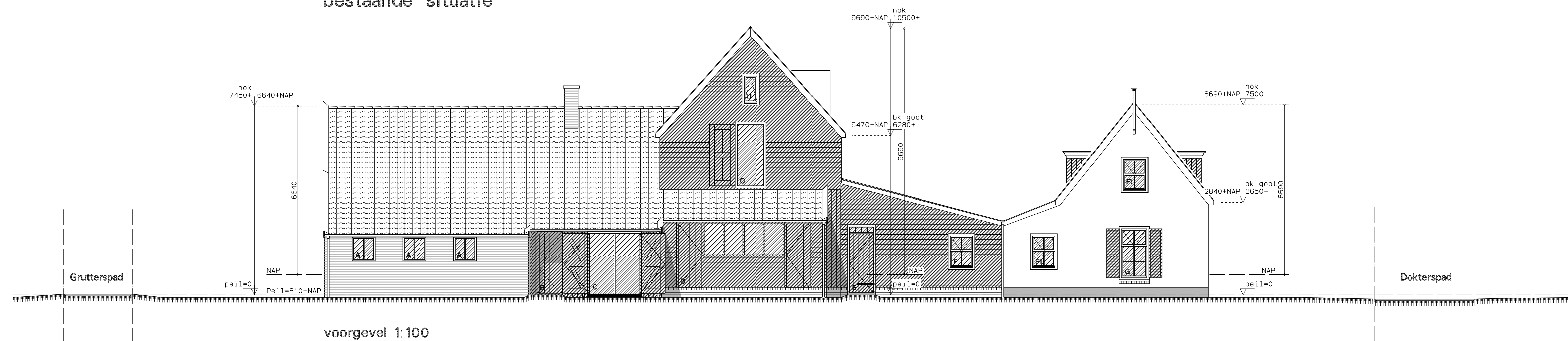
voorgevel 1:100 aanzicht vanaf Nieuwland bestaande situatie
