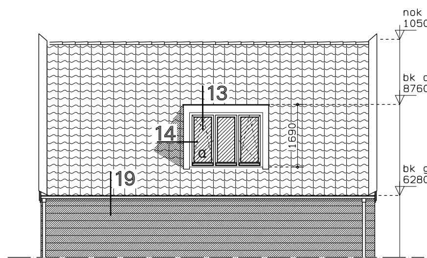
rechter zijgevel woning 2
