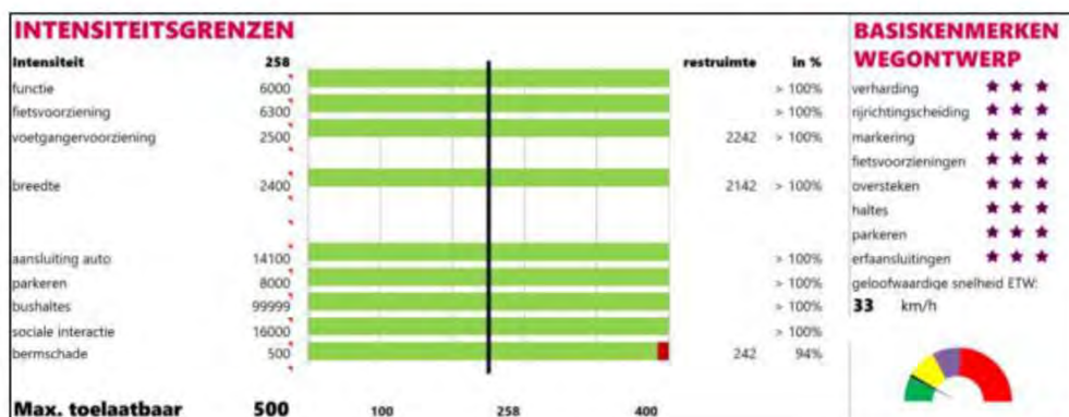
Figuur B2.2: Uitvoer Wegenscan Broekerveermeerdijk
