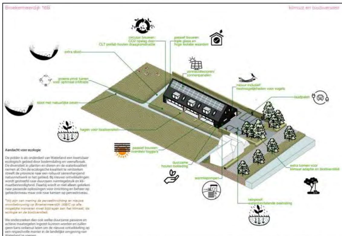
Figuur 5: Bovenaanzicht van de beoogde toekomstige situatie met de nieuw aan te leggen sloten met natuurlijke oever, aan te planten bomen en hagen, circulair, duurzaam en natuurinclusief bouwen en andere landschappelijke en milieubewuste keuzes.
